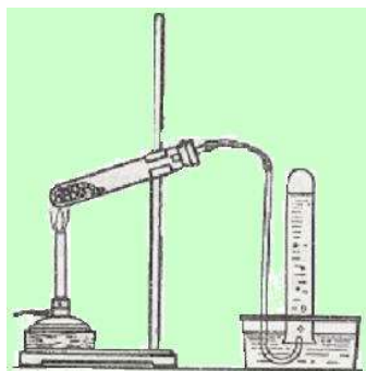
Рисунок 1 Прибор для получения метана.
